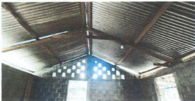
Foto 13: Cambio estructura de techo de madera a estructura metálica para la cocina.
